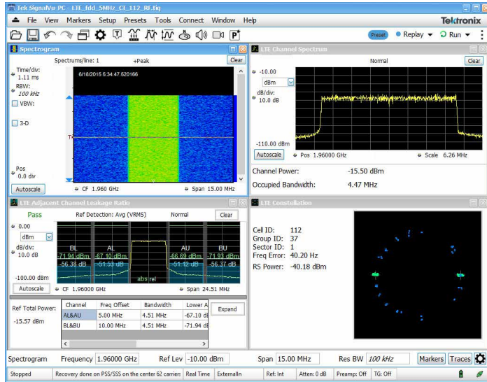
使用按钮预置和通过失败信息快速验证 LTE 基站发射机
