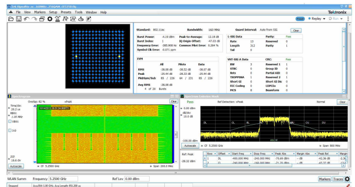
使用提供了频谱辐射模板、星座图和已解码突发信息的WLAN 预置简单地分析 WLAN 802.11ac 发射机。
